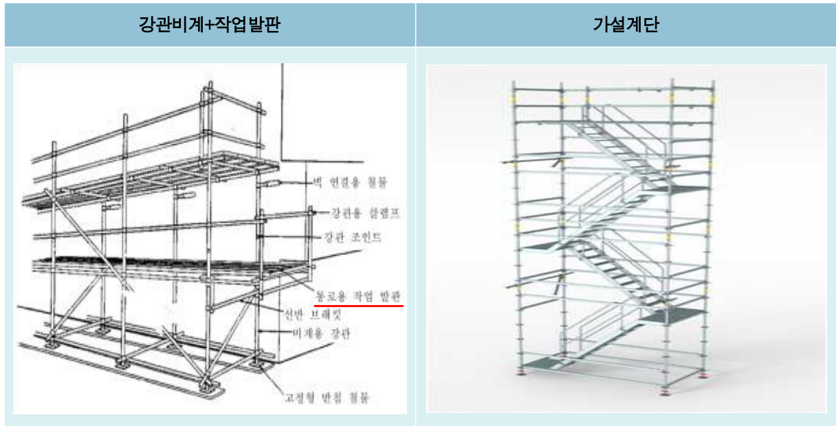
[그림 4] 강관비계 작업발판 및 가설계단
