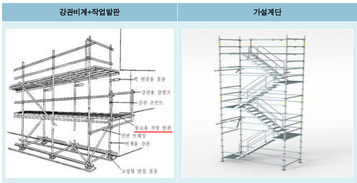
[그림 5] 강관비계 작업발판 및 가설계단
